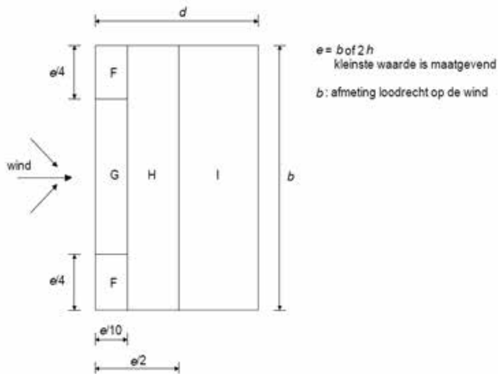
Figuur NB.5 – 7.6 — Zones bij platte daken – Gekromde of mansarde daken
